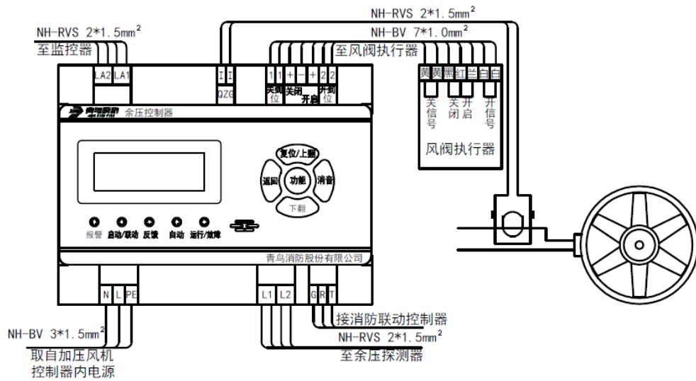
图 33 接线示意图
