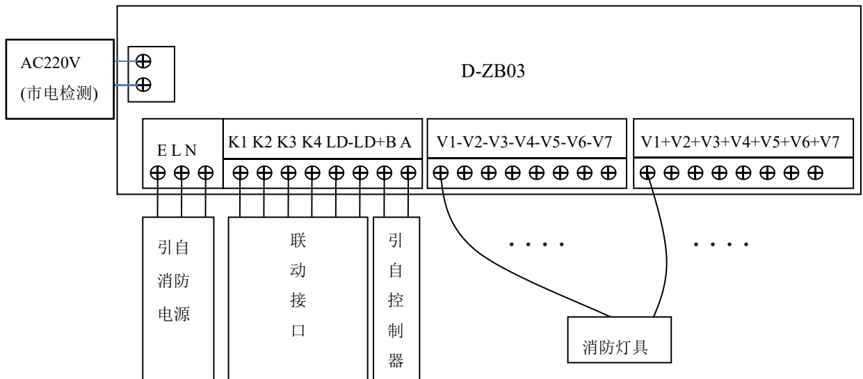
图 3.1 应急照明集中电源接线示意图
